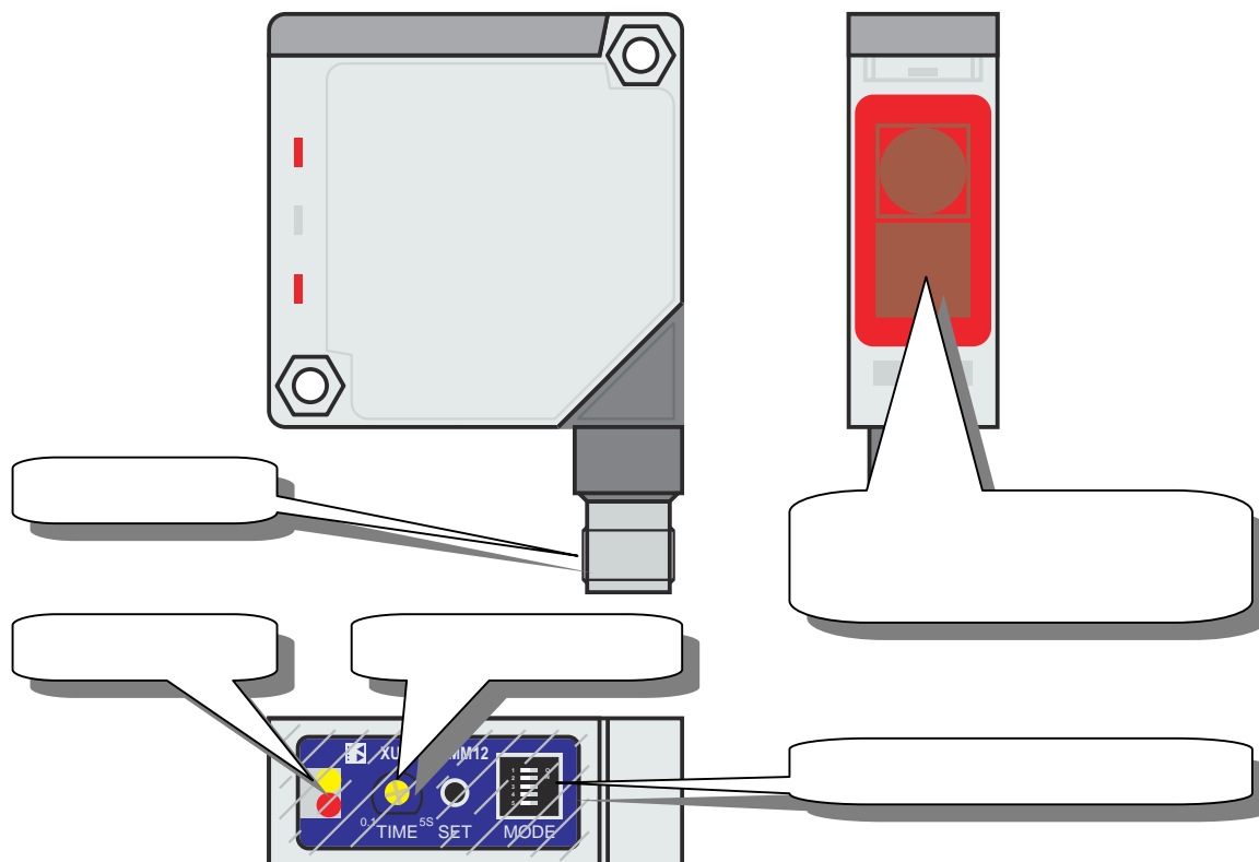
Détecteur optique type « reflex ».
